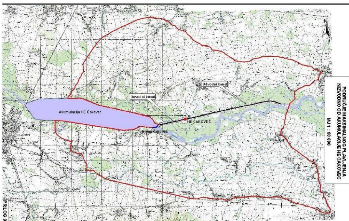
Slika 2: Područje maksimalnog plavljenja HE Čakovec Izvor podataka: HE Sjever
