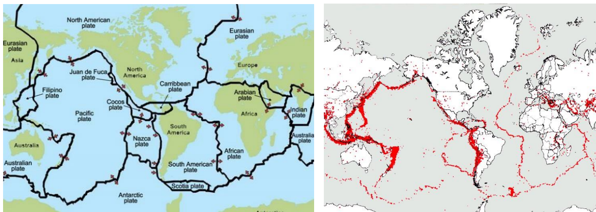
Slika 15: Tektonska građa Zemljine litosfere (lijevo) i Pregled epicentara potresa (desno)
